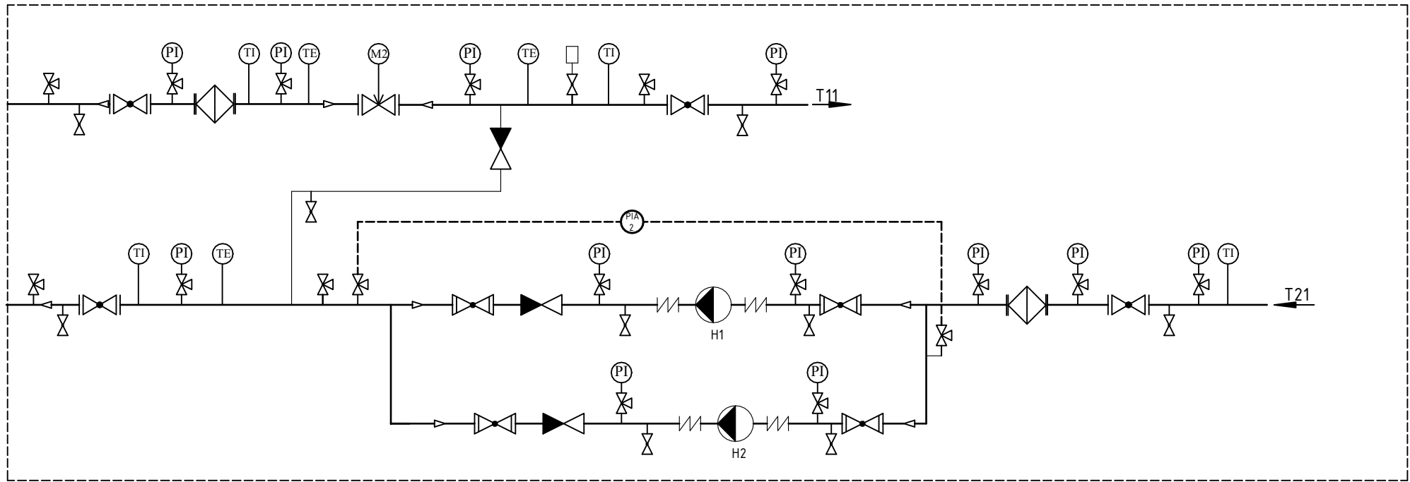
Рисунок 1 - Принципиальная схема блока "МЦЭ-БТПА-ТПА"
