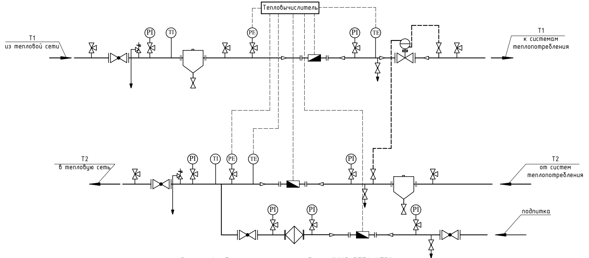
Рисунок 1 - Принципиальная схема блока "МЦЭ-БТПА-УТЭ"
