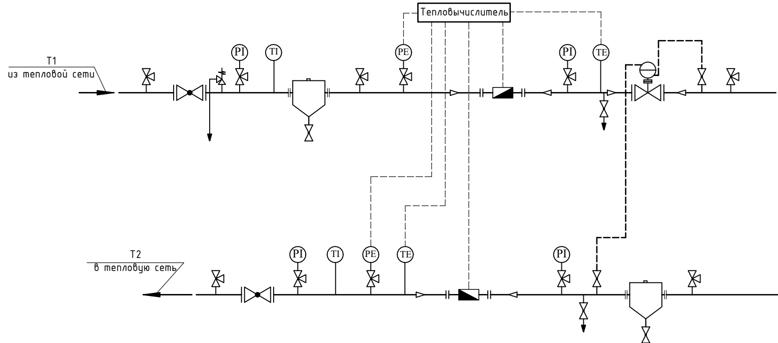
Рисунок 1 – Принципиальная схема блока “МЦЭ-БТПА-УТЭ”
